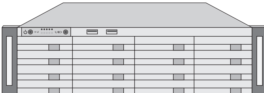
图1-1 TL-NVR616-256前面板示意图
