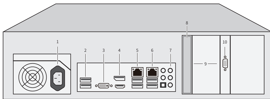
图1-3 TL-NVR616-256后面板示意图
